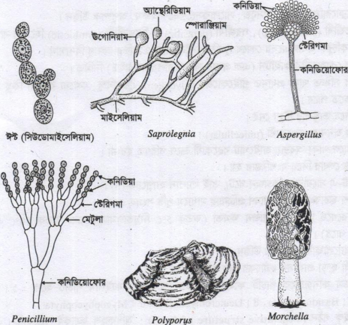
চিত্র ৫.৬ : কয়েকটি ছত্রাক। এর মধ্যে ইন্ট আগুবাঙ্কণিক, Polyporus ও Morchella খালি চোখে ভালো দেখা যায়; অন্য তিনটি সেমি আগুবাঙ্কণিক।
