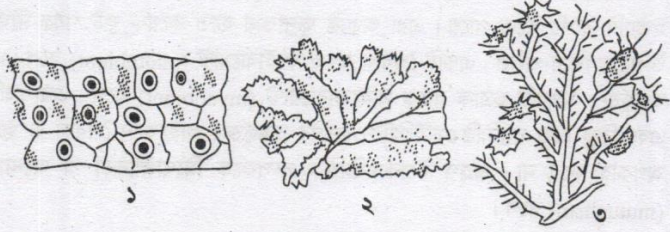
চিত্র ৫.১৩ : (১) ক্রাস্টোজ, (২) ফোলিয়োজ, (৩) ফ্রুটিকোজ লাইকেন
