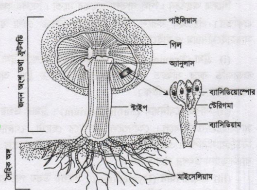
চিত্র ৫.৯ : Agaricus ছত্রাক-এর ফ্রুটবডি এবং অন্যান্য অংশ।
