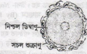
চিত্র ৫.২.১ : Fucus -এর উগ্যামাস জনন।
