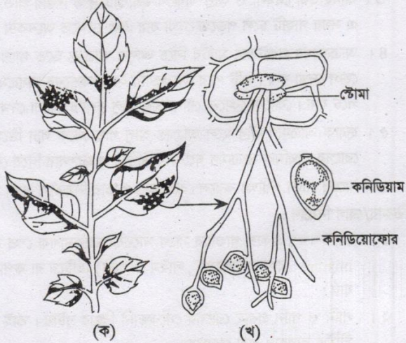
চিত্র ৫.১২ : Phytophthora infestans ছত্রাক (ক) আক্রান্ত আলু পাতা, (খ) কনিডিয়োফোর ও কনিডিয়া
