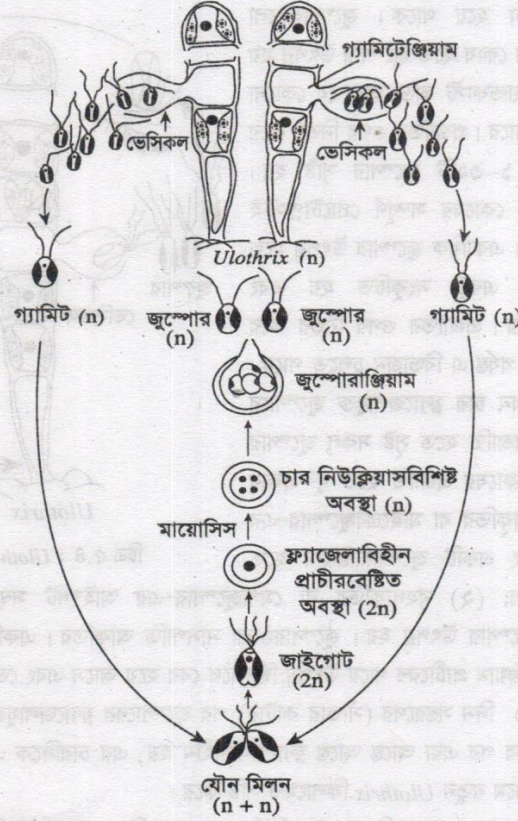
চিত্র ৫.৫ : Ulothrix-এর যৌন জনন।
