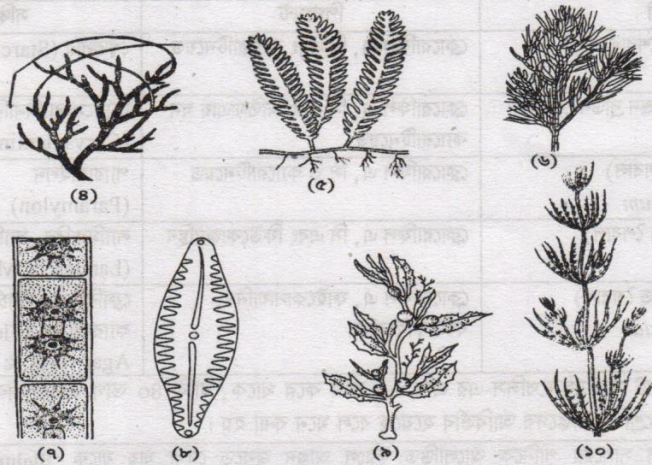
চিত্র ৫.১ : কয়েকটি শৈবাল : (১) Chlamydomonas ; (২) Volvox ; (৩) Spirogyra ; (৪) Chaetophora ; (৫) Caulerpa ; (৬) Polysiphonia (লোহিত শৈবাল); (৭) Zygnema ; (৮) Navicula (হলদে-সোনালী শৈবাল); (৯) Sargassum (বাদামি শৈবাল); (১০) Chara (৬, ৮ ও ৯নং ছাড়া অন্যগুলো সবুজ শৈবাল)।
