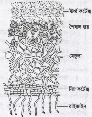
চিত্র ৫.১৪ : ফোলিয়োজ লাইকেনের অন্তর্গঠন
