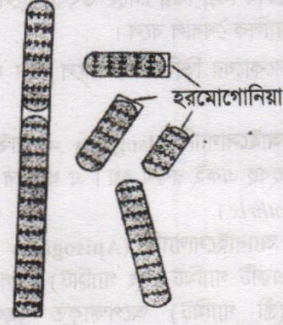
চিত্র ৫.১.১ : Oscillatoria শৈবালে খণ্ডায়ন
