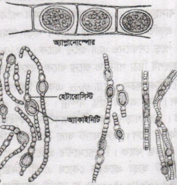
চিত্র ৫.১.২ : শৈবালে অ্যাপ্ল্যানোস্পোর, হেটারোসিস্ট ও অ্যাকাইনিটি
