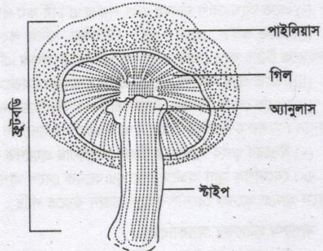
চিত্র ৫.১১.১: Agaricus ছত্রাক-এর ফুটবডি।
